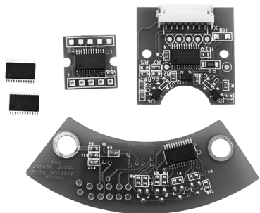
Fig. 10. MPS160 encoder.
