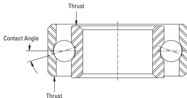
Fig. 15. Contact angle.
