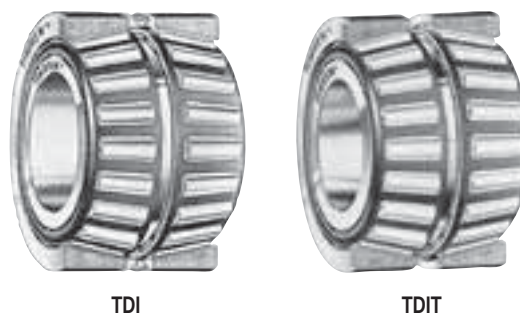
Рис. 4. Двухрядные подшипники с двойным внутренним кольцом.
