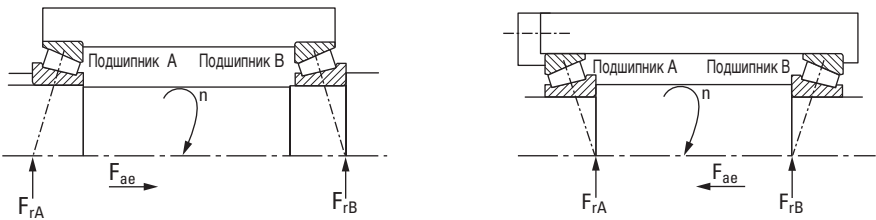
Конструкция (внешняя осевая сила F_{ae} , действующая на подшипник А)
