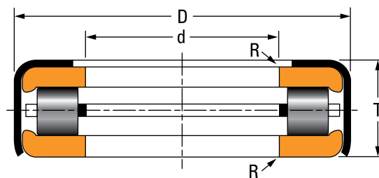
Fig. 79. Type TTSP.
