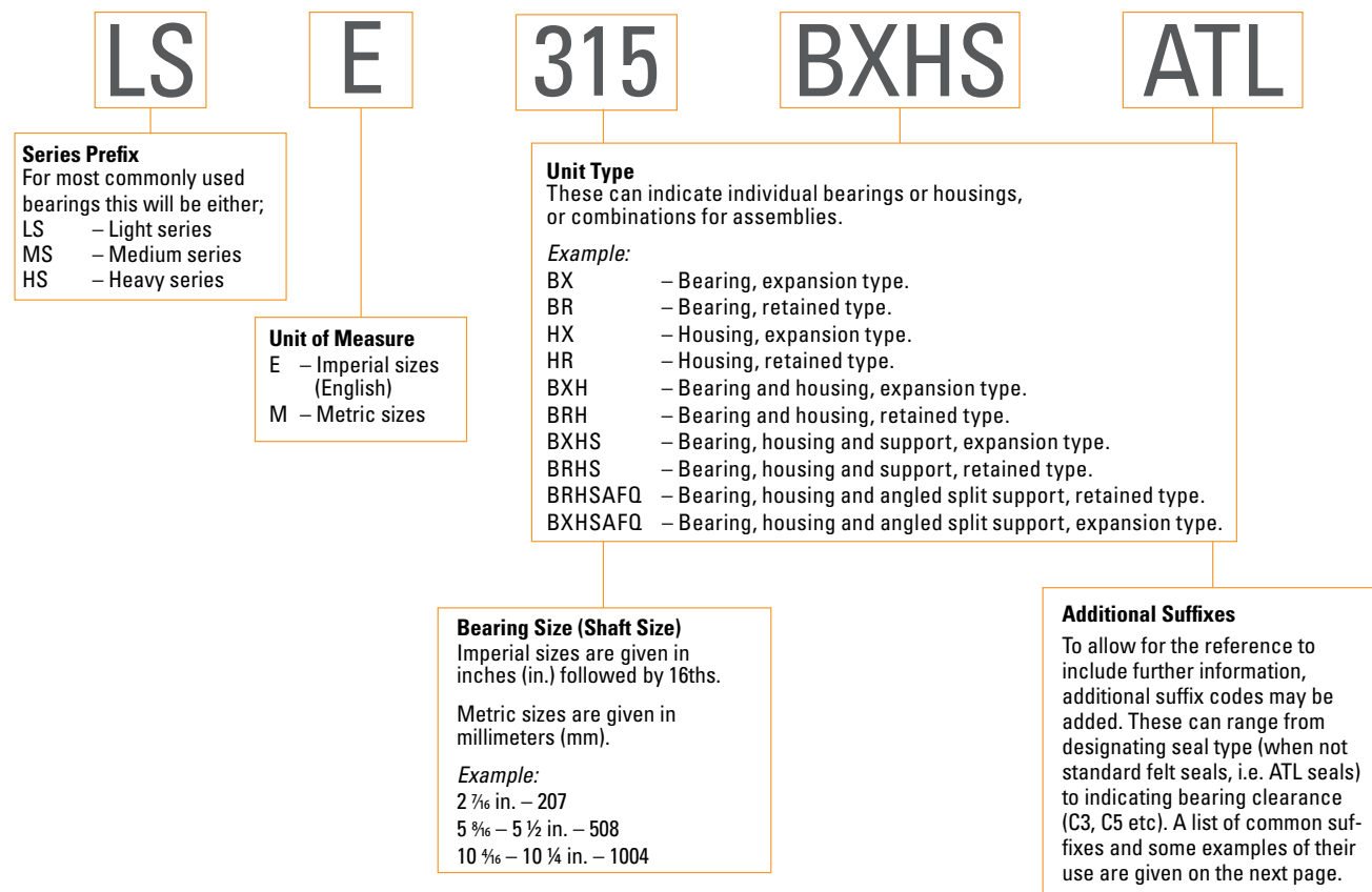
Fig. 3. Nomenclature.
