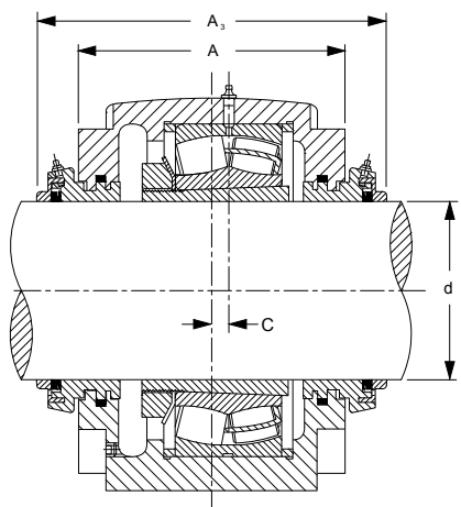
Таконитовое уплотнение
