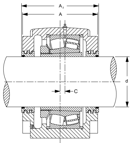
Лабиринтное уплотнение
