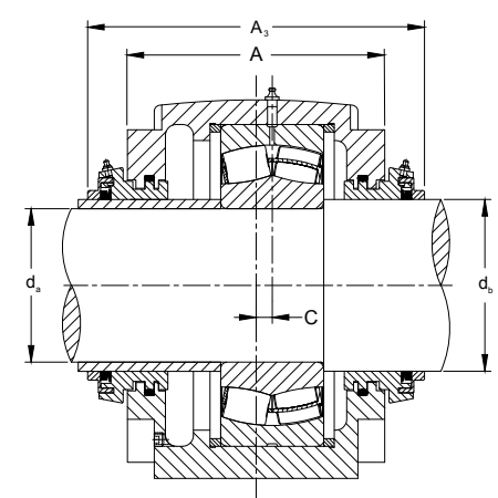
Таконитовое уплотнение
