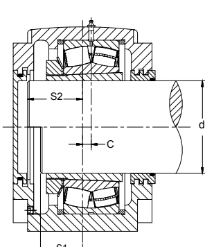
Подшипник с коническим отверстием на фиксирующей втулке Торцевая крышка/Лабиринтное уплотнение
