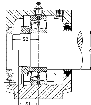
Подшипник с цилиндрическим отверстием Торцевая крышка/Двухманжетное уплотнение
