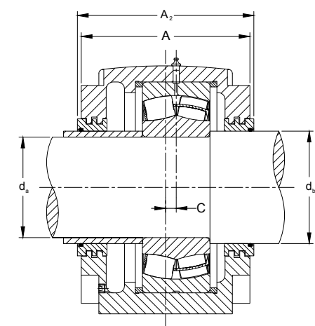
Лабиринтное уплотнение
