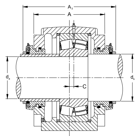
Таконитовое уплотнение
