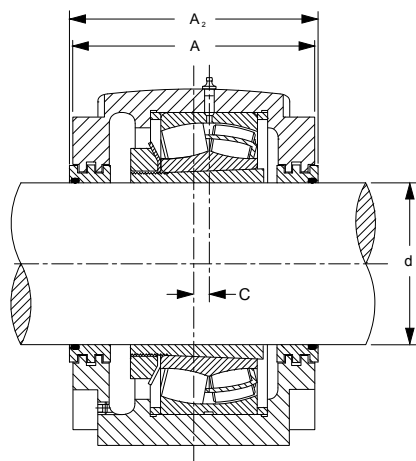
Лабиринтное уплотнение
