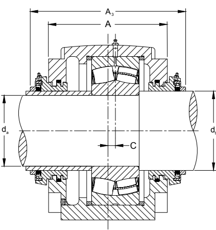
Таконитовое уплотнение
