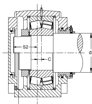
Подшипник с цилиндрическим отверстием Торцевая крышка/Таконитовое уплотнение
