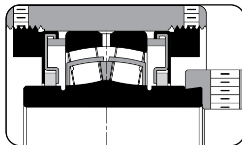
Fig. 14. T seal.
